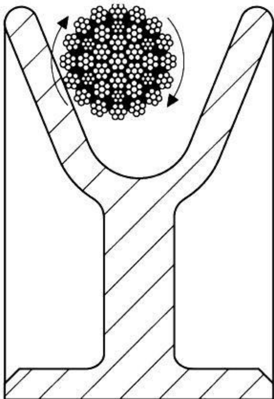
Рисунок А.5 - Кручение каната на ребрах блока
