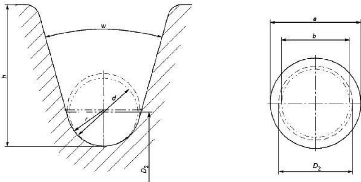
Рисунок А.3 - Канавка блока
